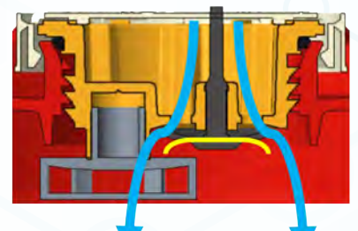
Automatyczne przewietrzanie
