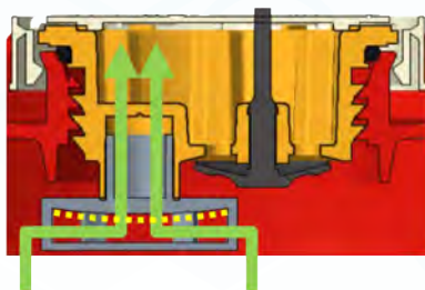
Automatyczny odpowietrznik
